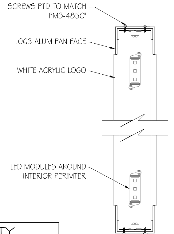
SECTION A-A SCALE: 1 1/2" = 1'-0"
