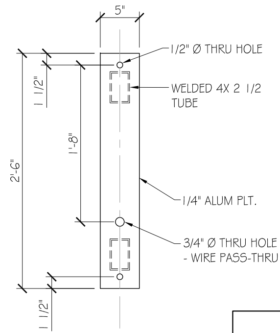
MTG. PLATE SCALE: 1" = 1'-0"
