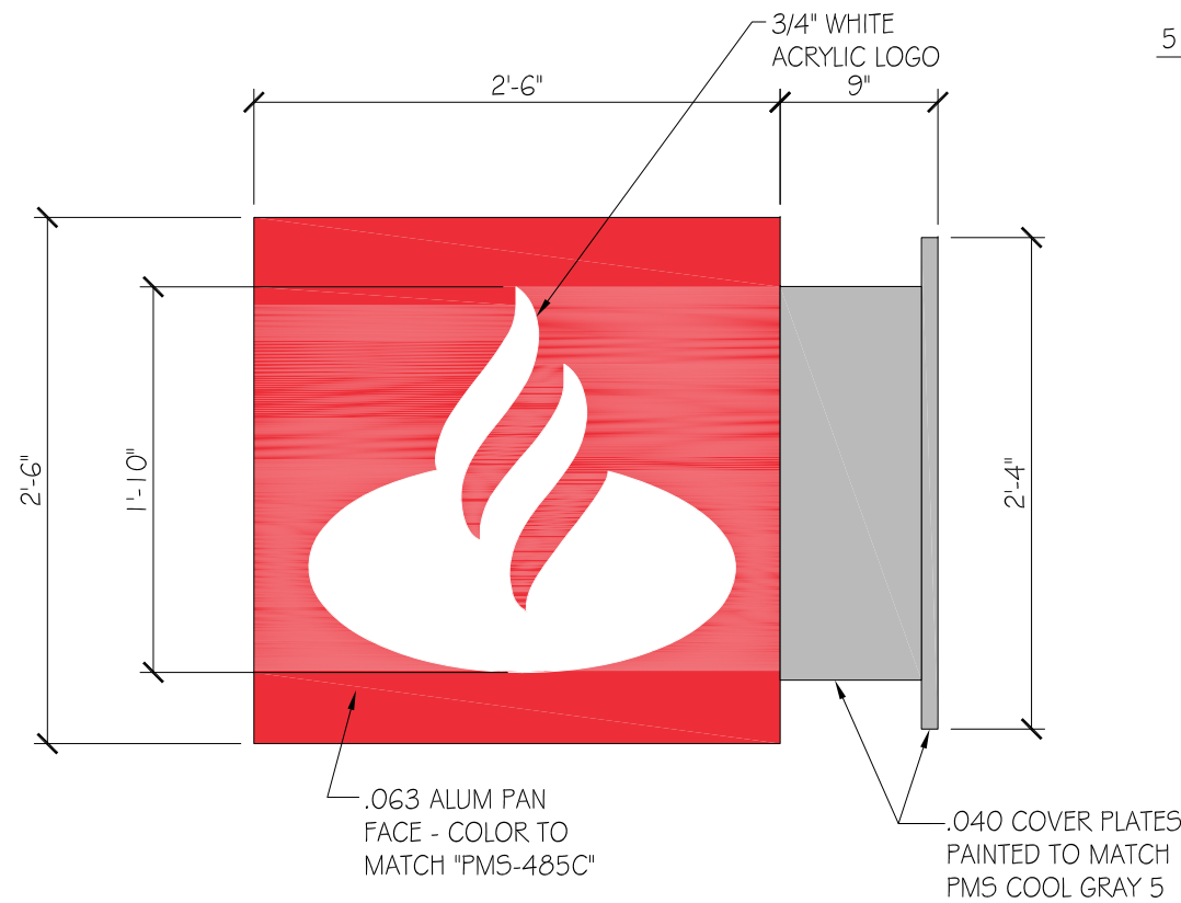
ELEVATION SCALE: 1" = 1'-0"
