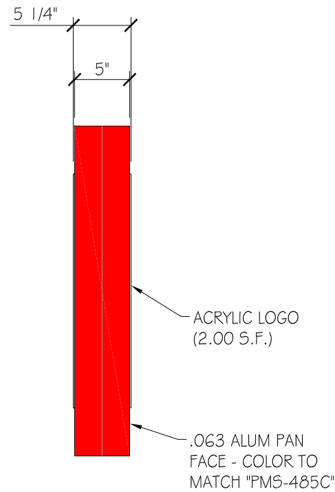
END VIEW SCALE: 1" = 1'-0"
