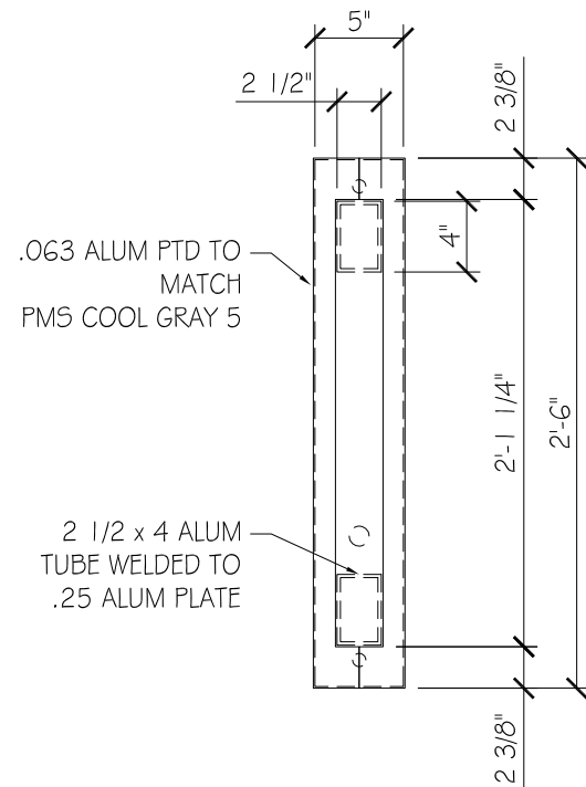
ESCUTCHEON PLATE SCALE: 1" = 1'-0"
