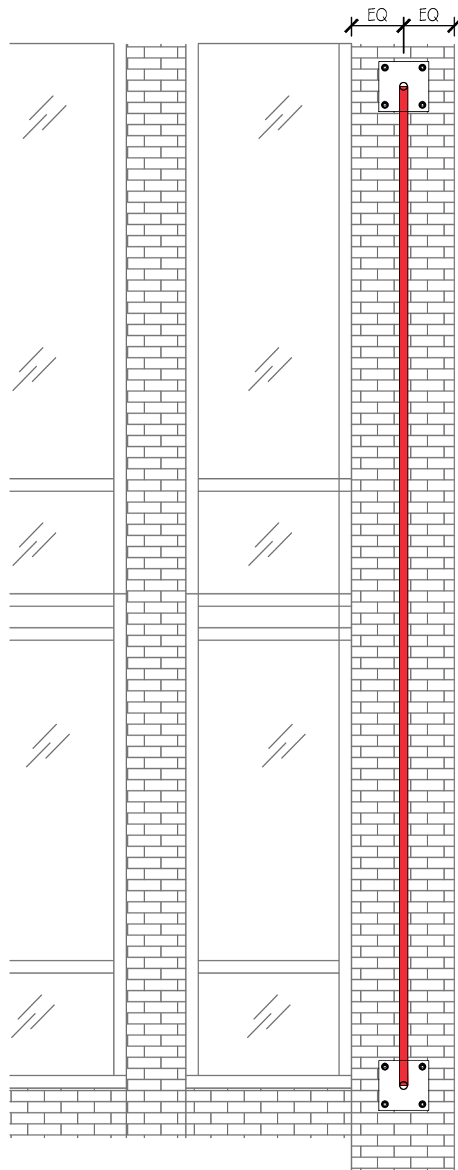
PARTIAL FRONT ELEV. SCALE: 3/8" = 1'-0"
